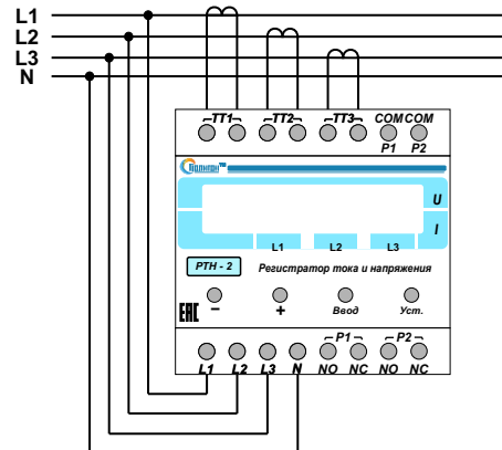
Рис.7. Схема подключения РТН-2 к сети.
