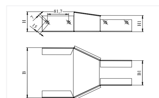
Лотки монтажные глухие типа КШВГ, тип перехода - центральный. Применяются для лотков типа ЛМГ; ЛМГЗ.
