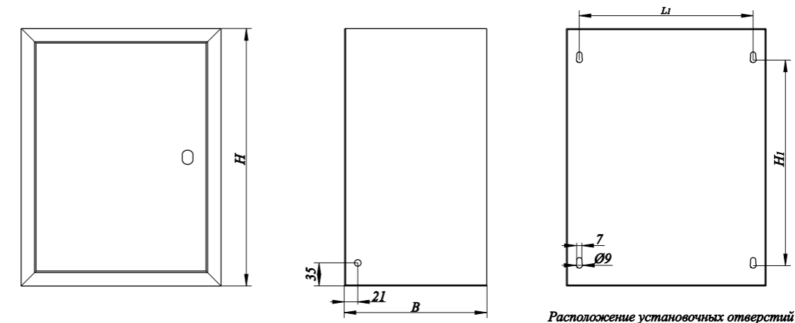
Расположение установочных отверстий
