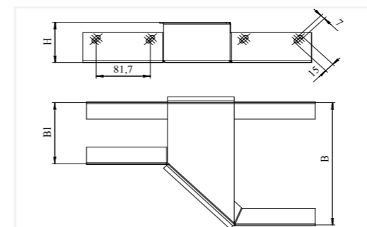
Лотки монтажные глухие типа КШГл, тип перехода - левый. Применяются для лотков типа ЛМГ; ЛМГЗ.
