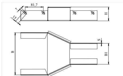
Лотки монтажные глухие типа КШГ, тип перехода - центральный. Применяются для лотков типа ЛМГ; ЛМГЗ.
