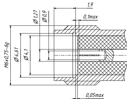
Соединители тип IX, вар. 1 и тип SMA (розетка)
