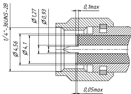
Соединители тип IX, вар. 1 и тип SMA (вилка)
