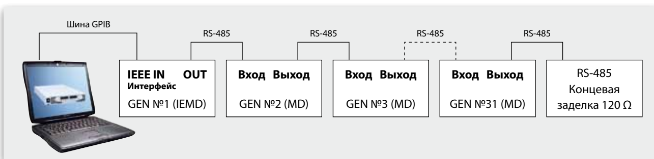
Конфигурация многоканального интерфейса источников питания
