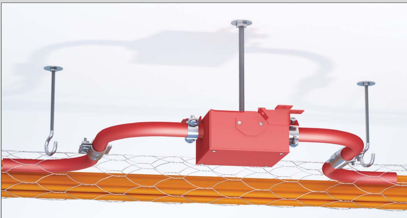
Рис. 21. Пример монтажа ОКЛ «СПЕЦКАБЛАЙН-К2» с монтажной коробкой
