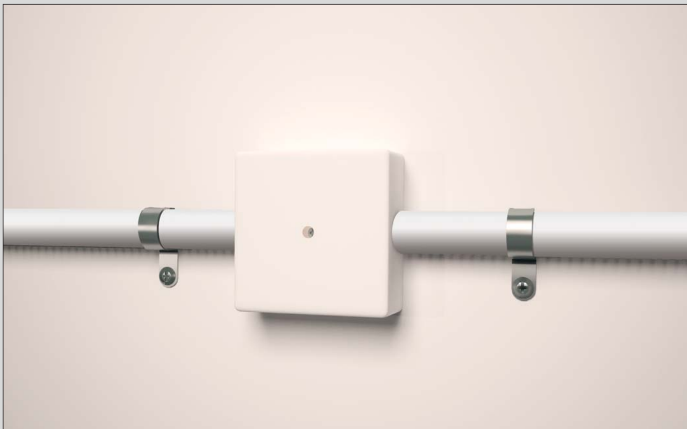
Рис. 10. ОКЛ «СПЕЦКАБЛАЙН-ГФ(ГЛ)20»
