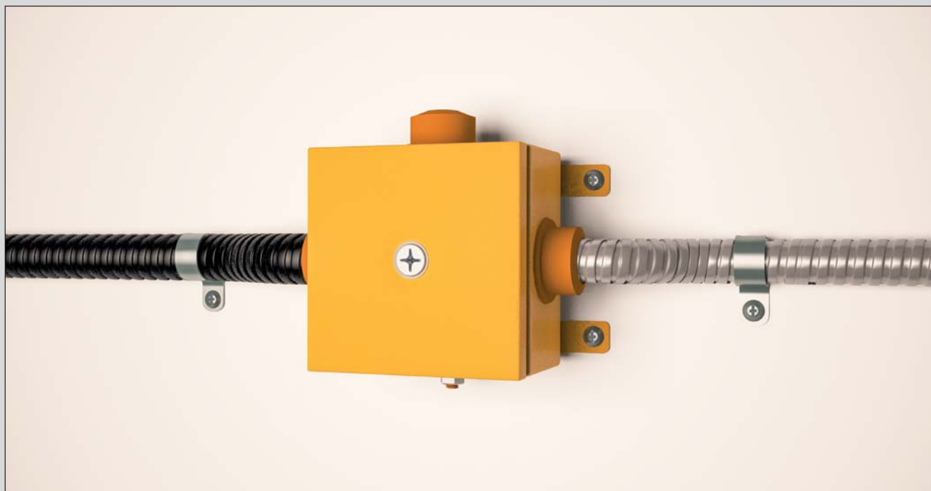
Рис. 7. ОКЛ «СПЕЦКАБЛАЙН-КиТ» в металлическом рукаве
