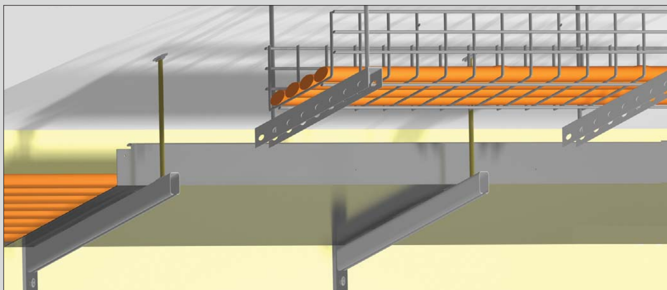
Рис. 20. ОКЛ «СПЕЦКАБЛАЙН-0»
