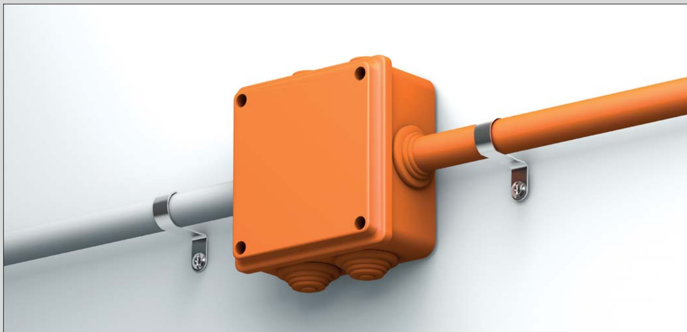
Рис. 5. ОКЛ «СПЕЦКАБЛАЙН-КиТ» в гладкой трубе
