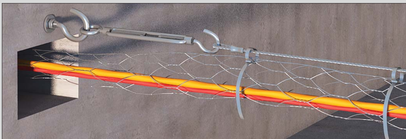
Рис. 11. ОКЛ «СПЕЦКАБЛАЙН-Тр»
