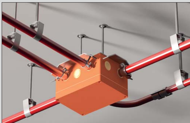
Рис. 24. Пластиковые огнестойкие коробки KSK
