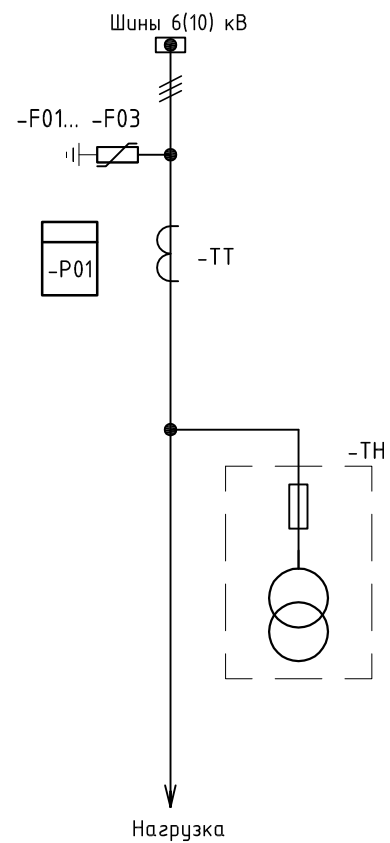
Схема главных цепей
