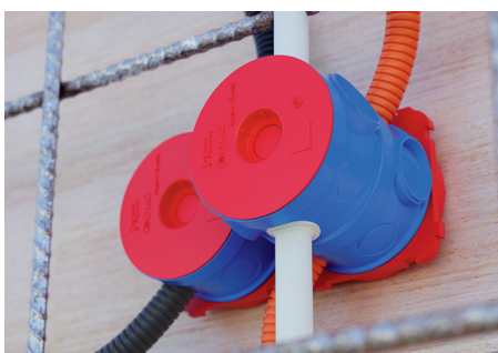
Сборка коробки и укладка бетонной смеси
