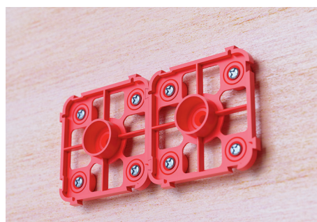
Монтаж крышки к опалубке
