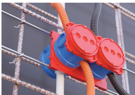
Монтаж коробок к арматурному каркасу
