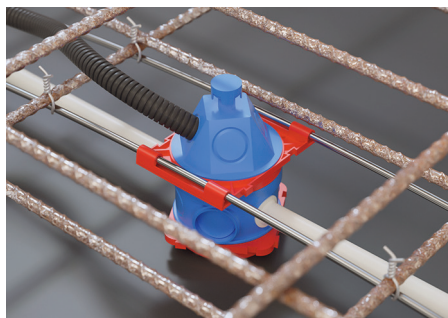
Монтаж коробки к арматурному каркасу, укладка бетонной смеси
