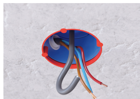
Демонтаж опалубки, протяжка кабеля, установка крюка
