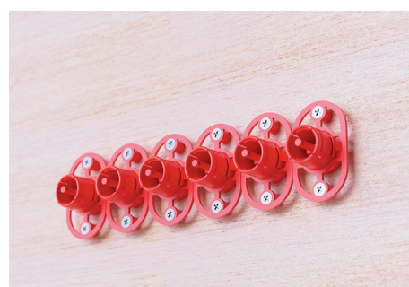
Монтаж втулки к опалубке
