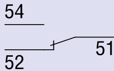
Схема электрическая принципиальная независимого расцепителя
