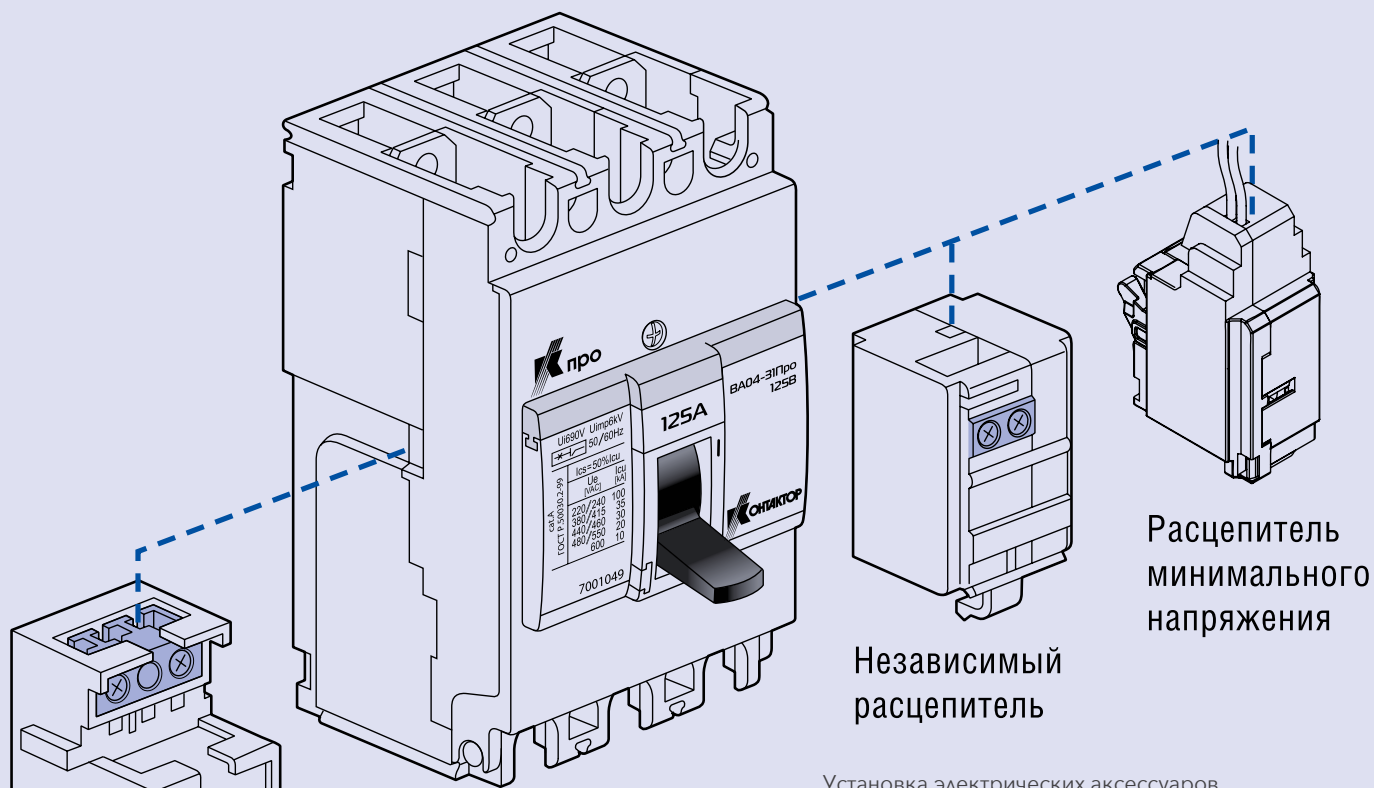
Установка электрических аксессуаров
