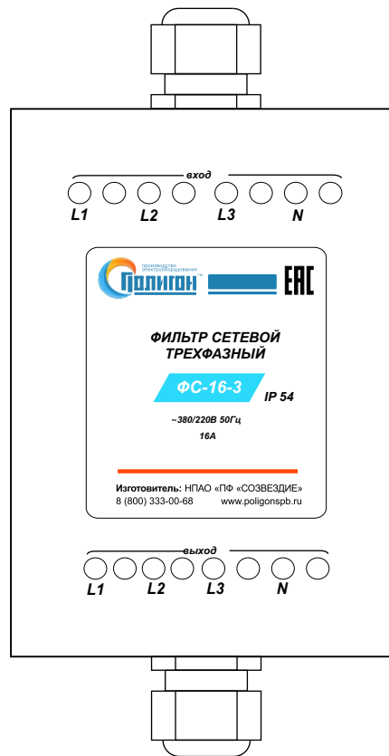
Рис.1. Порядок подключения фильтра FC-16-3 IP54.
