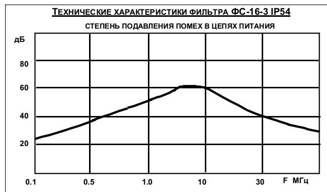
Рис.2. График АЧХ фильтра FC-16-3 IP54 .
