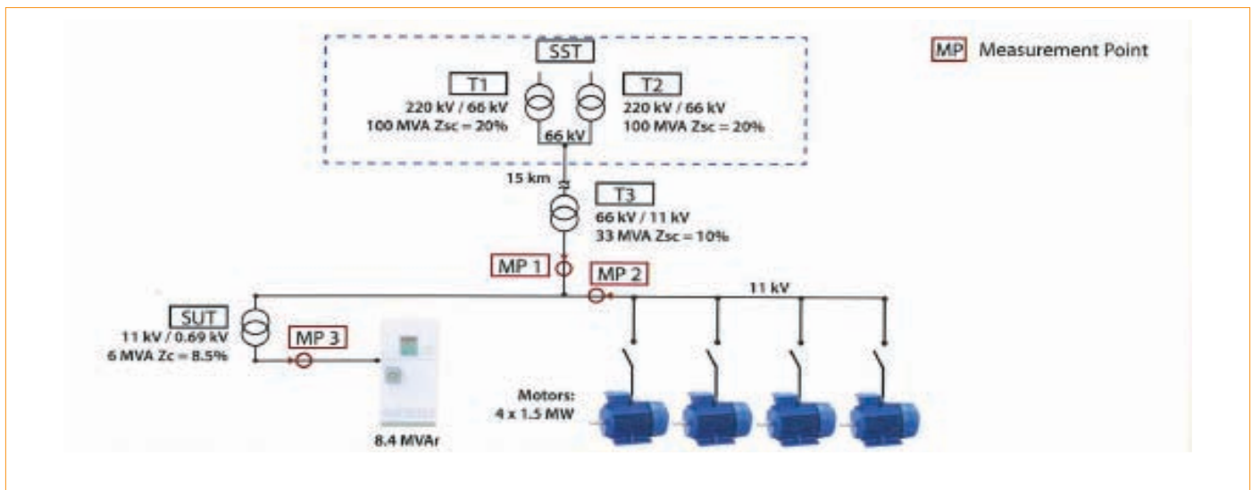
Actual Electrical Diagram – 11 kV & Network
