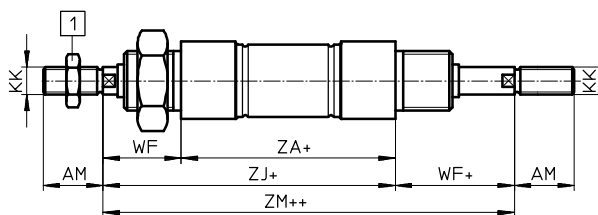
S2 – Сквозной шток
