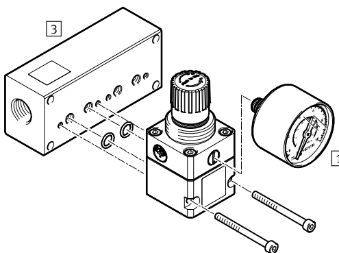
Прецизионный регулятор давления LRP-7.0-6
