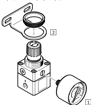
Прецизионный регулятор давления LRP-1/8-6
