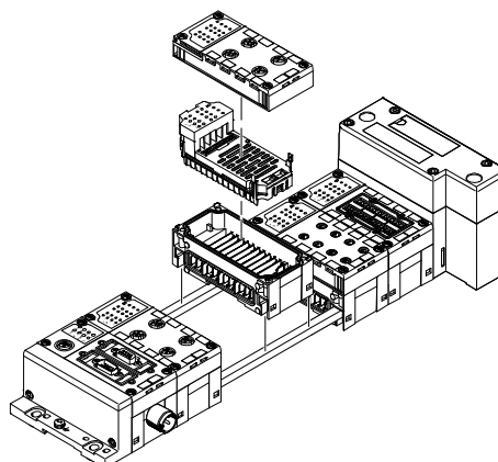
Модульная структура для электрической периферии CPX
