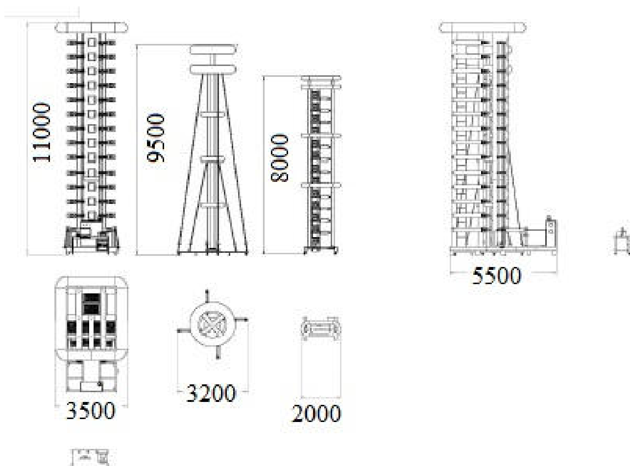
Габаритные размеры элементов ГИН
