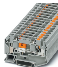
Гибридные (винт - Push-in) 6 мм 2
