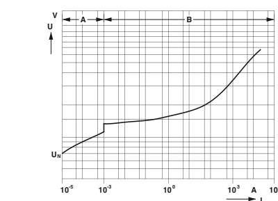
ВАХ металлооксидных варисторов Обозначения:
