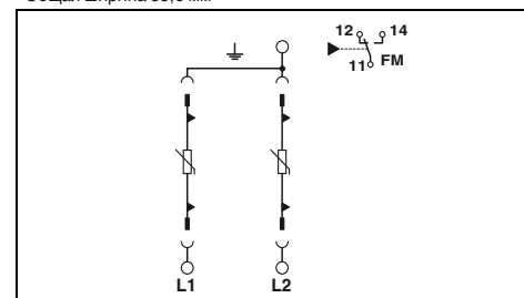
3-проводная система, L1, L2, G, 3-фазный треугольник с заземлением угловой точки
