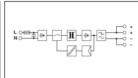
Источник питания, 1 AC, 24 В DC, 60 Вт NEC, класс 2
