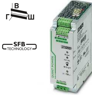
Преобразователь постоянного тока, 60 – 72 В DC / 24 В DC, 10 А
