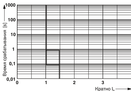
Характеристика срабатывания
