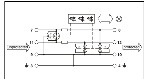
2 проводника, с общим опорным потенциалом, подключение 9/10, прямое заземление, например, для двоичных сигналов
