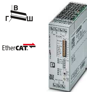
Источник бесперебойного питания, 24 В DC / 24 В DC, 40 А, EC
