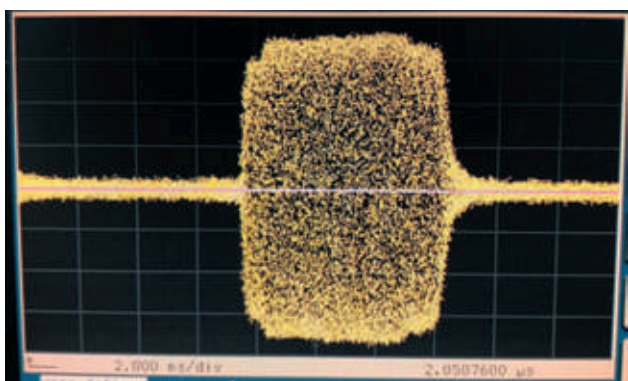
Рисунок 19: Пример ИМ сигнала генератора MMSG40, 38.8 ГГц, 15 нс период, 7 нс период.
