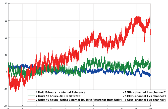
Рисунок 4: Типичное значение ошибки фазы между каналами двух приборов во временной области
