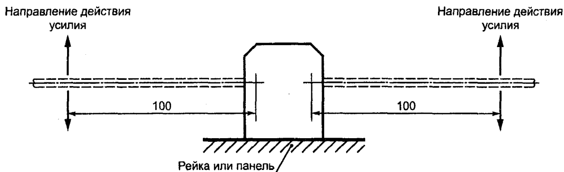
Рисунок 1 — Установка для испытания
